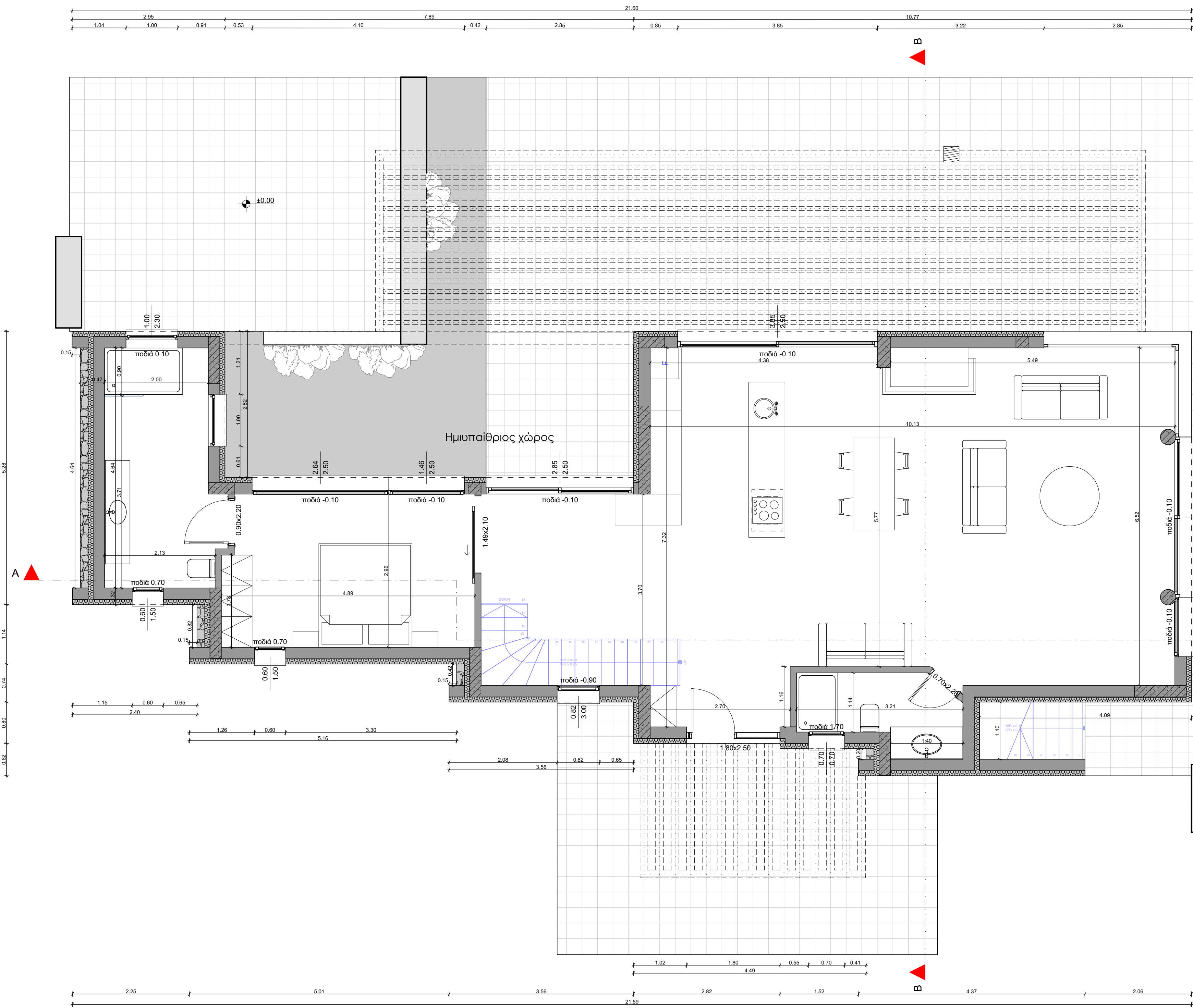
κάτοψη ορόφου Εολ = 73.57 τ.μ.
