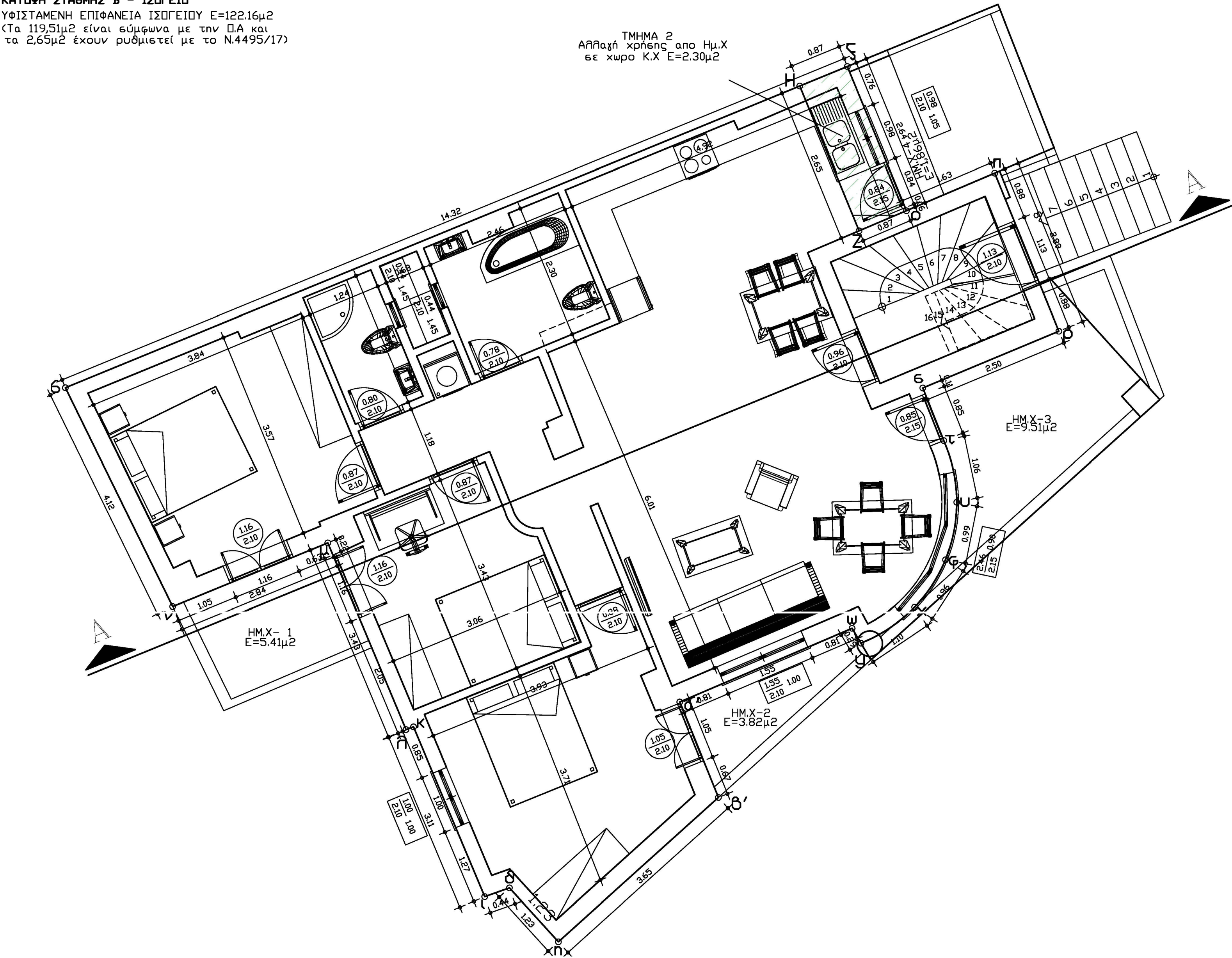
ΚΑΤΩΨΗ ΙΣΟΓΕΙΟΥ
